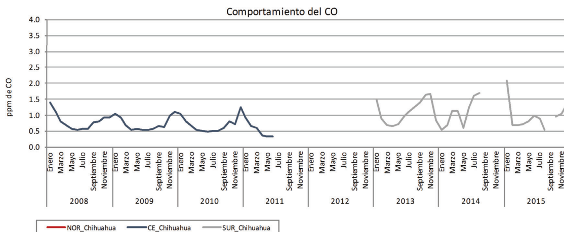
Figura 22d. Comportamiento de CO durante los meses del año en la Ciudad de Chihuahua.
