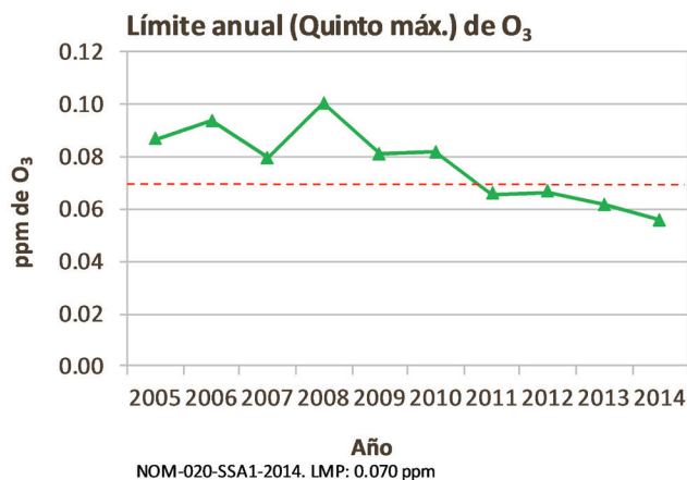
Figura 14d. O 3 . Límite anual (quinto máx. de las concentraciones diarias de los promedios. móviles de 8 h) para Ciudad Juárez.
