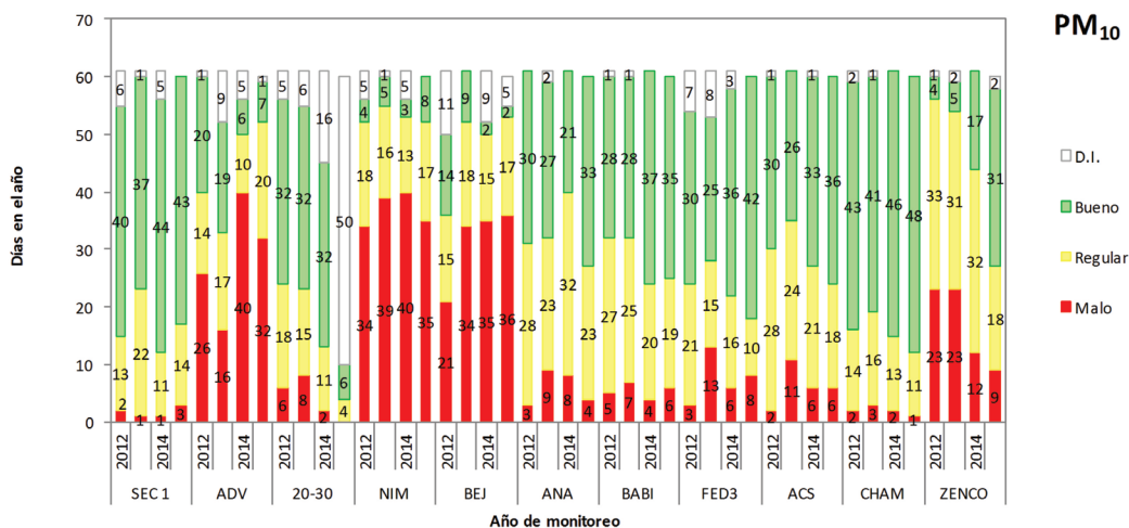
Figura 16b. Distribución de los días con calidad del aire buena, regular y mala para PM_{10} en las diferentes estaciones de monitoreo atmosférico de Cd. Juárez.
