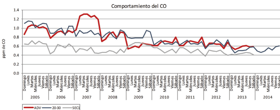
Figura 25c. Comportamiento de CO durante los días de la semana en Ciudad Juárez.
