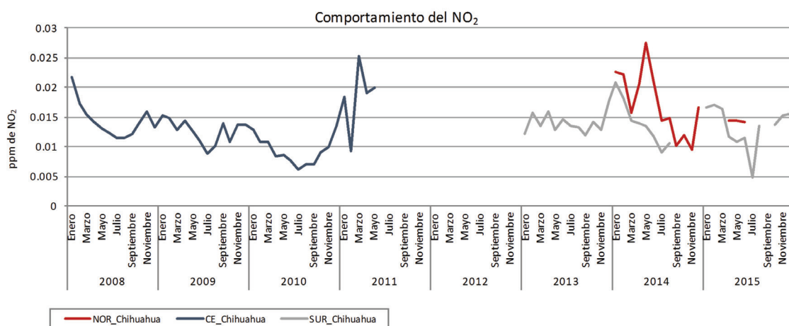
Figura 22e. Comportamiento de NO 2 durante los meses del año en la Ciudad de Chihuahua.
