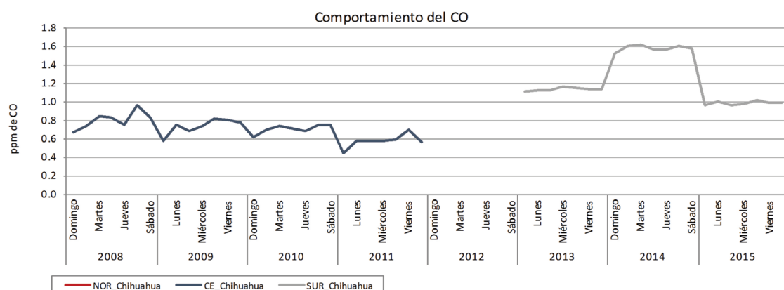
Figura 24d. Comportamiento de CO durante los días de la semana en la Ciudad de Chihuahua.
