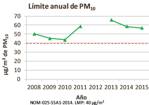
Figura 12a. PM_{10} . Límite anual (promedio anual de los promedios de 24 h) para la Ciudad de Chihuahua.
