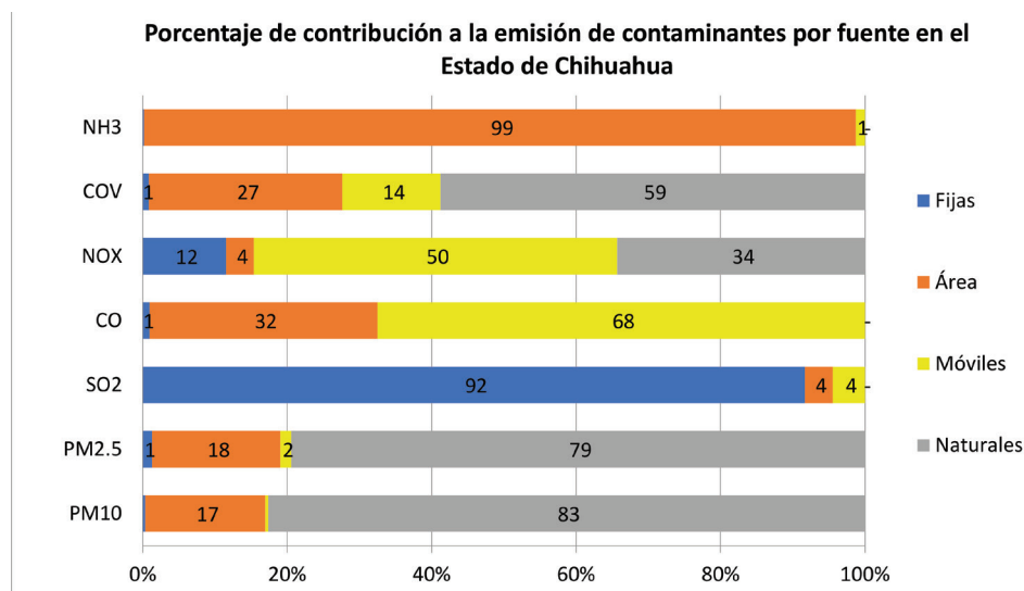
Figura 28. Porcentaje de emisión por fuente en el Estado de Chihuahua.
