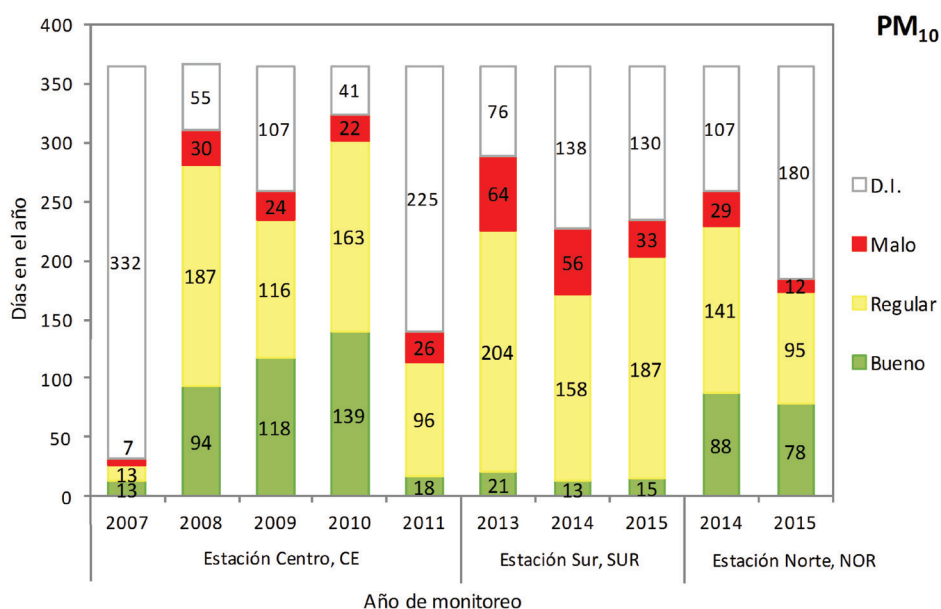
Figura 16a. Distribución de los días con calidad del aire buena, regular y mala para PM_{10} en las diferentes estaciones de monitoreo atmosférico de la Ciudad de Chihuahua.
