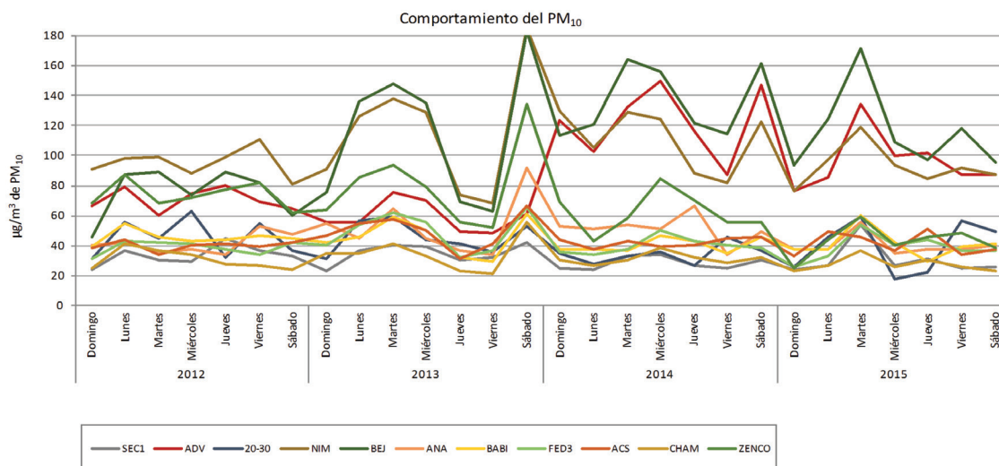
Figura 25a. Comportamiento de \text{PM}_{10} durante los días de la semana en Ciudad Juárez.
