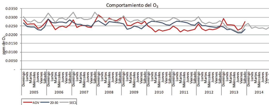
Figura 25b. Comportamiento de O_3 durante los días de la semana en Ciudad Juárez.
