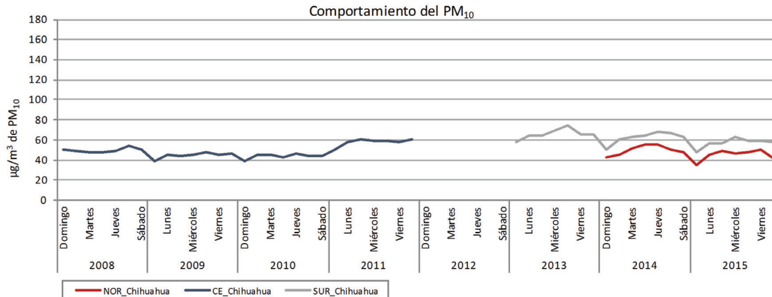
Figura 24a. Comportamiento de PM_{10} durante los días de la semana en la Ciudad de Chihuahua.
