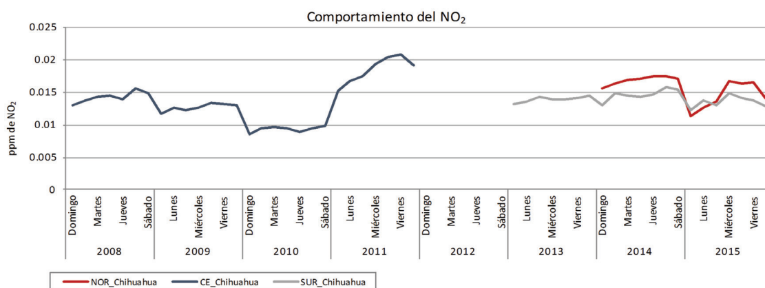
Figura 24e. Comportamiento de \text{NO}_2 durante los días de la semana en la Ciudad de Chihuahua.
