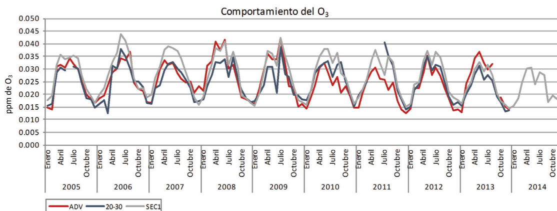
Figura 23b. Comportamiento de O_3 durante los meses del año en Ciudad Juárez.
