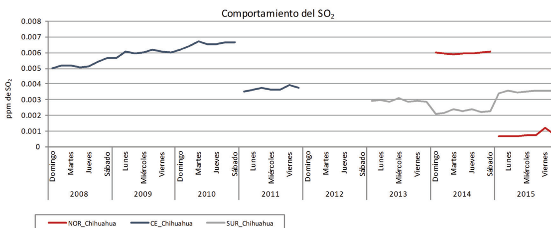
Figura 24f. Comportamiento de \text{SO}_2 durante los días de la semana en la Ciudad de Chihuahua.
