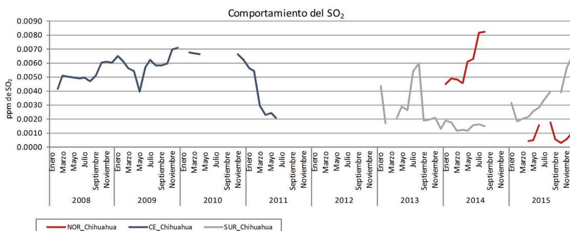
Figura 22f. Comportamiento de SO 2 durante los meses del año en la Ciudad de Chihuahua.
