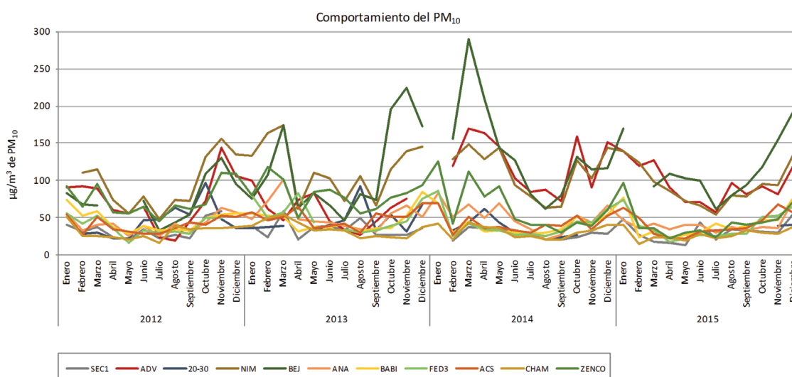
Figura 23a. Comportamiento de PM_{10} durante los meses del año en Ciudad Juárez.
