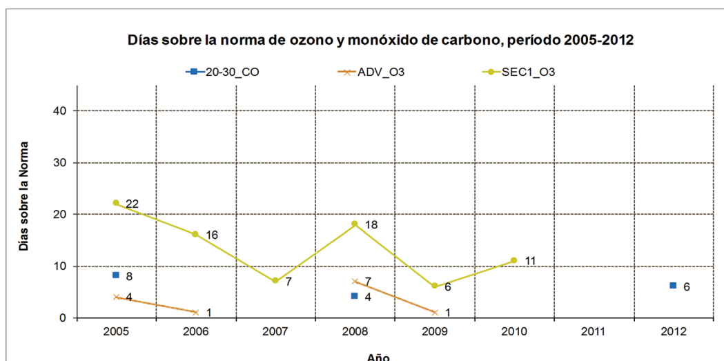
Figura 10c. Historial de Ciudad Juárez sobre el cumplimiento de la NOM para O 3 y CO.
