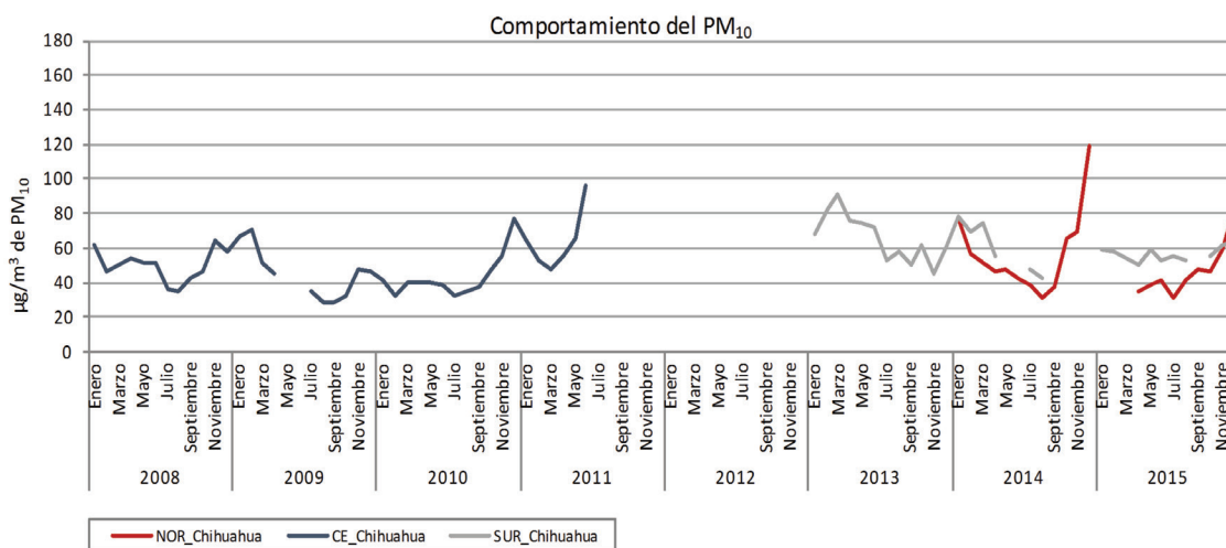
Figura 22a. Comportamiento de PM 10 durante los meses del año en la Ciudad de Chihuahua.
