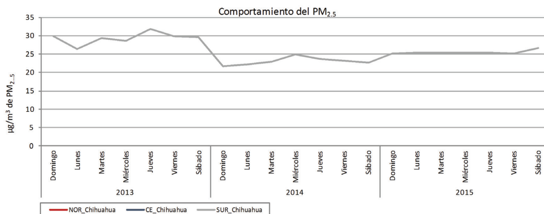
Figura 24b. Comportamiento de PM_{2.5} durante los días de la semana en la Ciudad de Chihuahua.
