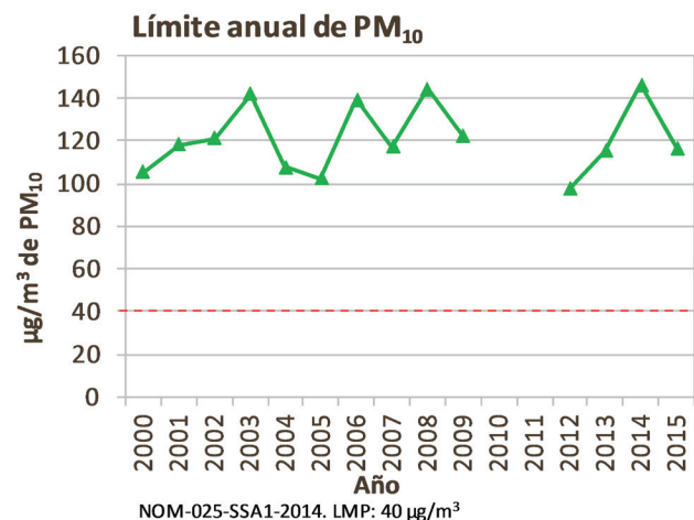
Figura 12c. PM_{10} . Límite anual (promedio anual de los promedios de 24 h) para Ciudad Juárez.
