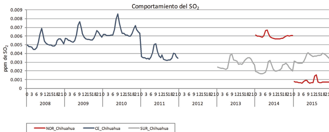
Figura 26f. Comportamiento de \text{SO}_2 durante las horas del día en la Ciudad de Chihuahua.
