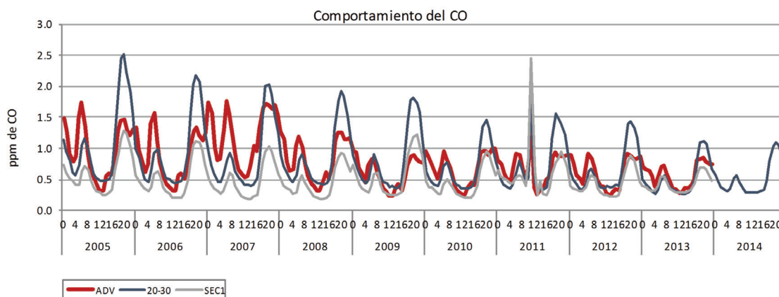
Figura 27b. Comportamiento de \text{CO} durante las horas del día para Cd. Juárez.
