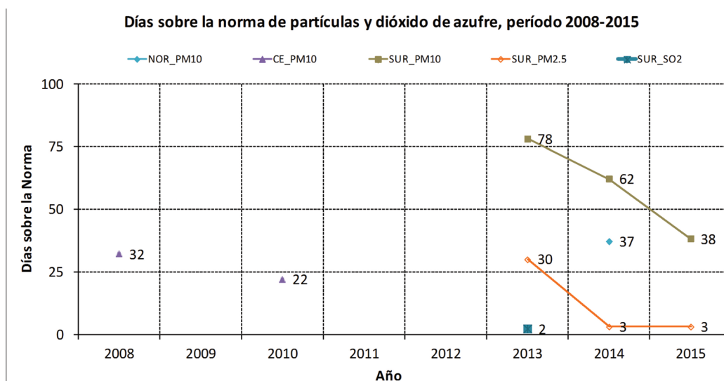
Figura 10a. Historial de la Ciudad de Chihuahua sobre el cumplimiento de la NOM para PM_{10} , PM_{2.5} y SO_2 .
