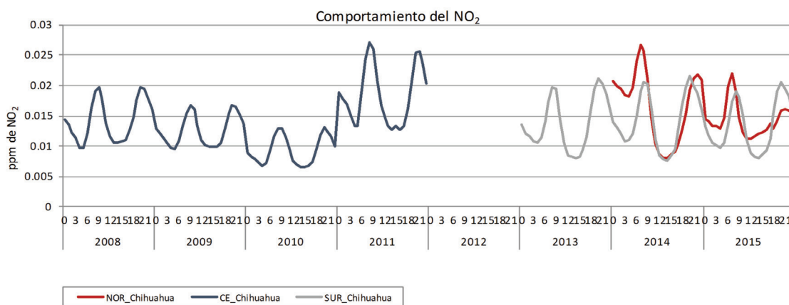
Figura 26e. Comportamiento de NO_2 durante las horas del día en la Ciudad de Chihuahua.
