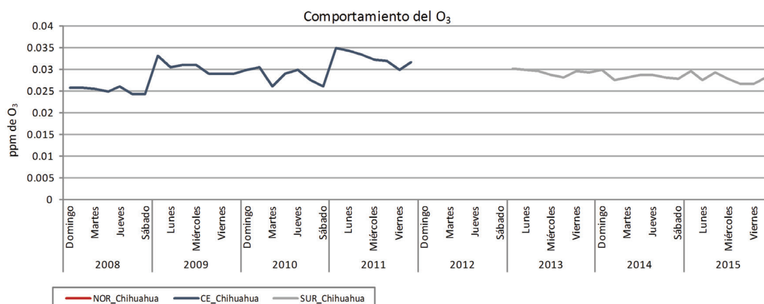
Figura 24c. Comportamiento de O_3 durante los días de la semana en la Ciudad de Chihuahua.
