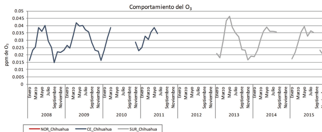
Figura 22c. Comportamiento de O 3 durante los meses del año en la Ciudad de Chihuahua.
