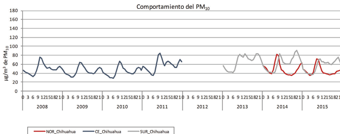
Figura 26a. Comportamiento de PM_{10} durante las horas del día en la Ciudad de Chihuahua.
