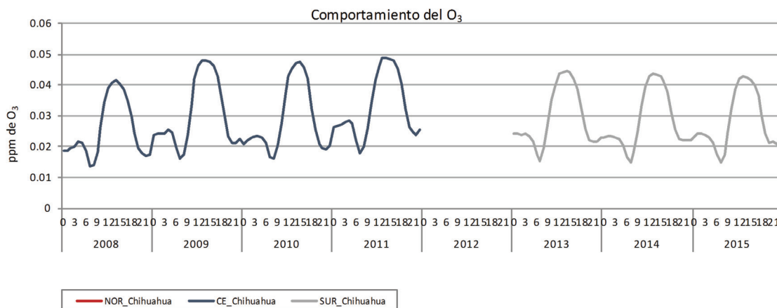
Figura 26c. Comportamiento de O_3 durante las horas del día en la Ciudad de Chihuahua.
