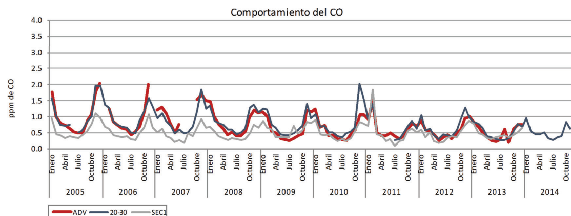
Figura 23c. Comportamiento de CO durante los meses del año para Cd. Juárez.
