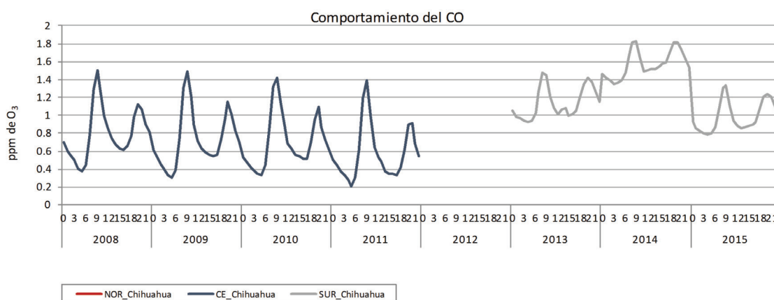
Figura 26d. Comportamiento de CO durante las horas del día en la Ciudad de Chihuahua.
