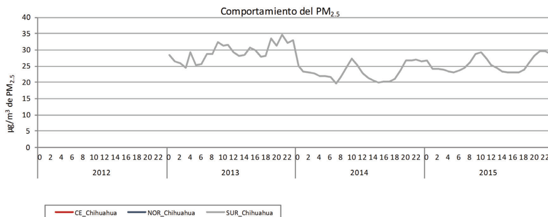
Figura 26b. Comportamiento de PM_{2.5} durante las horas del día en la Ciudad de Chihuahua.
