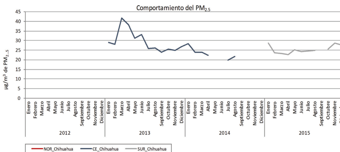
Figura 22b. Comportamiento de PM 2.5 durante los meses del año en la Ciudad de Chihuahua.
