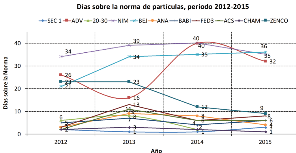
Figura 10b. Historial de Ciudad Juárez sobre el cumplimiento de la NOM para PM_{10} .
