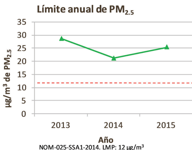
Figura 13a. PM 2.5 . Límite anual (promedio anual de los promedios de 24 h) para Chihuahua.
