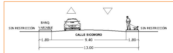
Figura 46. Calle Sicomoro. Sección actual PDU 20410.
