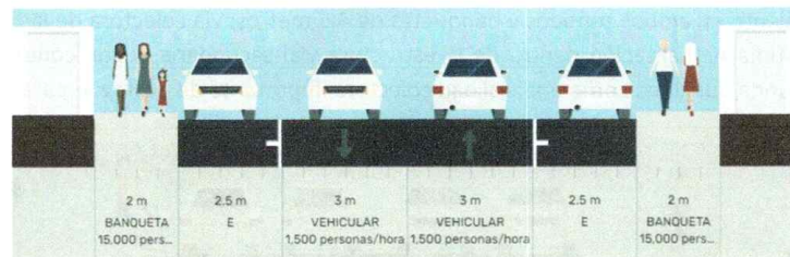
Imagen 29. Sección Vial SA-017A. Fuente PDU 2040 séptima actualización
