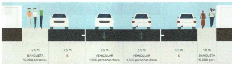
Imagen 29. Sección Vial SA-004. Fuente PDU 2040 séptima actualización
