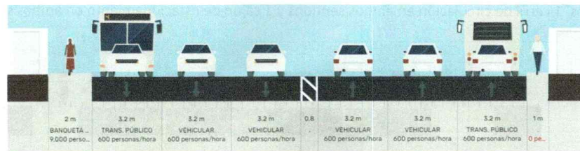
Imagen 29. Sección Vial PA-099C. Fuente PDU 2040 séptima actualización
