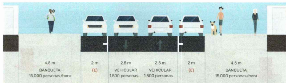
Imagen 45. Sección Vial calle Elía según PDU Séptima Actualización
