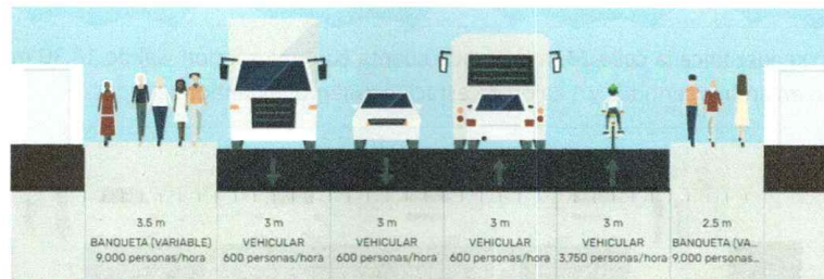
Imagen 29. Sección Vial PA-125D. Fuente PDU 2040 séptima actualización
