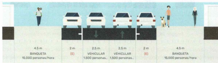
Imagen 29. Sección Vial SA-082. Fuente PDU 2040 séptima actualización
