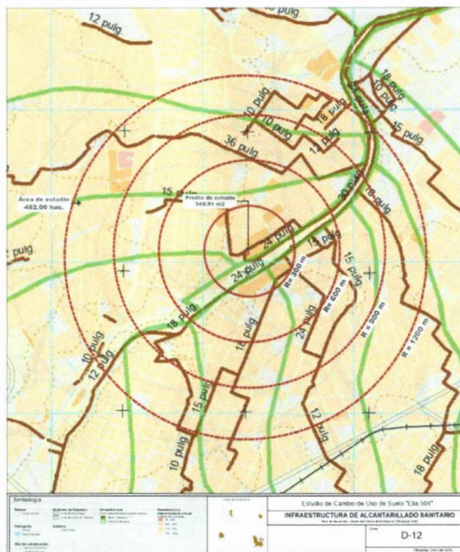
Imagen 33. Infraestructura de alcantarillado en la zona, fuente: PDU 2040
